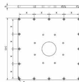
Nr. 16 Tasselli chimici CONTROPIASTRA Z2
