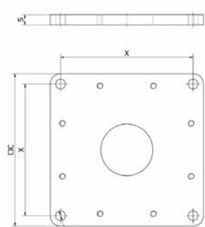
Nr. 4 Tasselli chimici CONTROPIASTRA R - S
