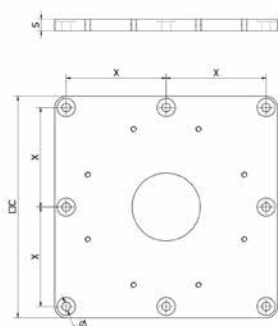
Nr. 8 Tasselli chimici CONTROPIASTRA T
